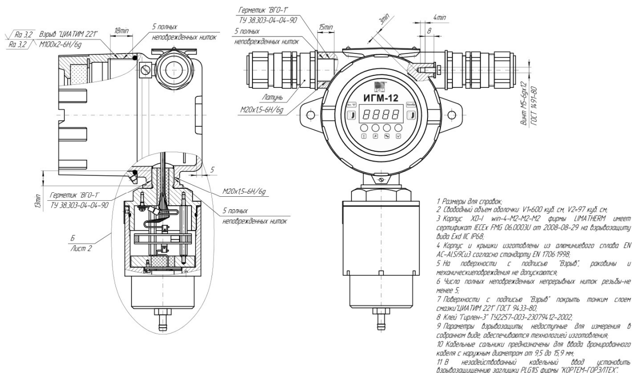
Рисунок В.1 – Чертеж средств взрывозащиты газоанализатора ИГМ-12.
