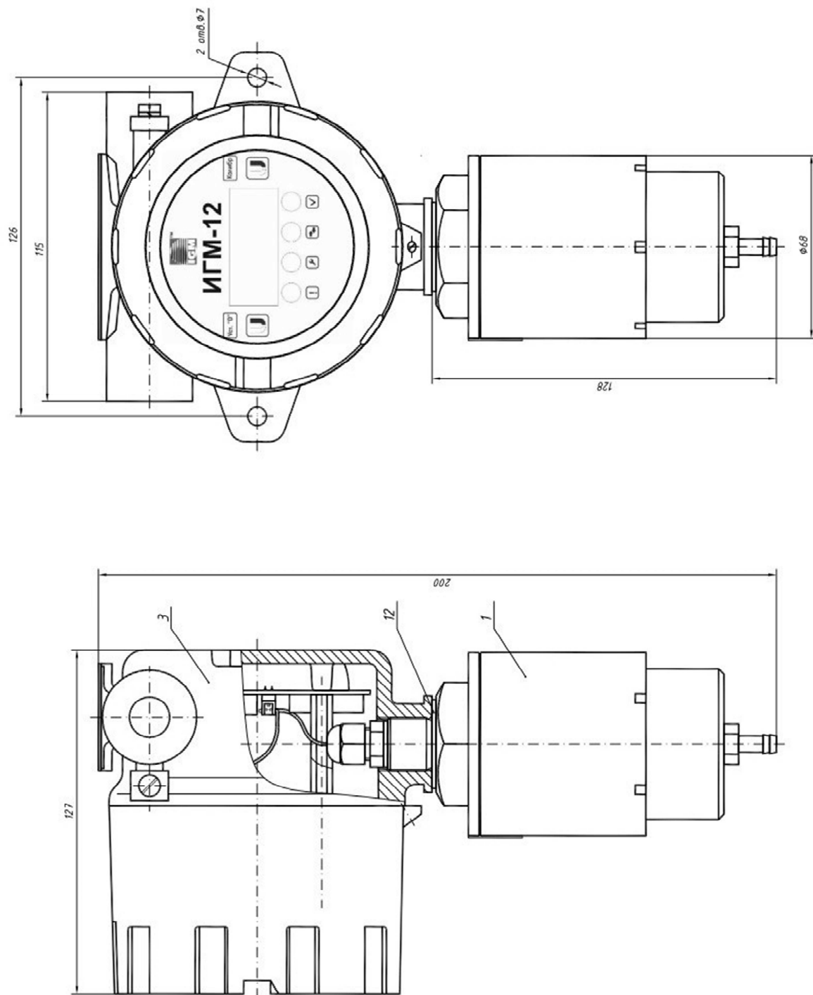
Рисунок Г.1 - Габаритный чертеж ИГМ-12.
