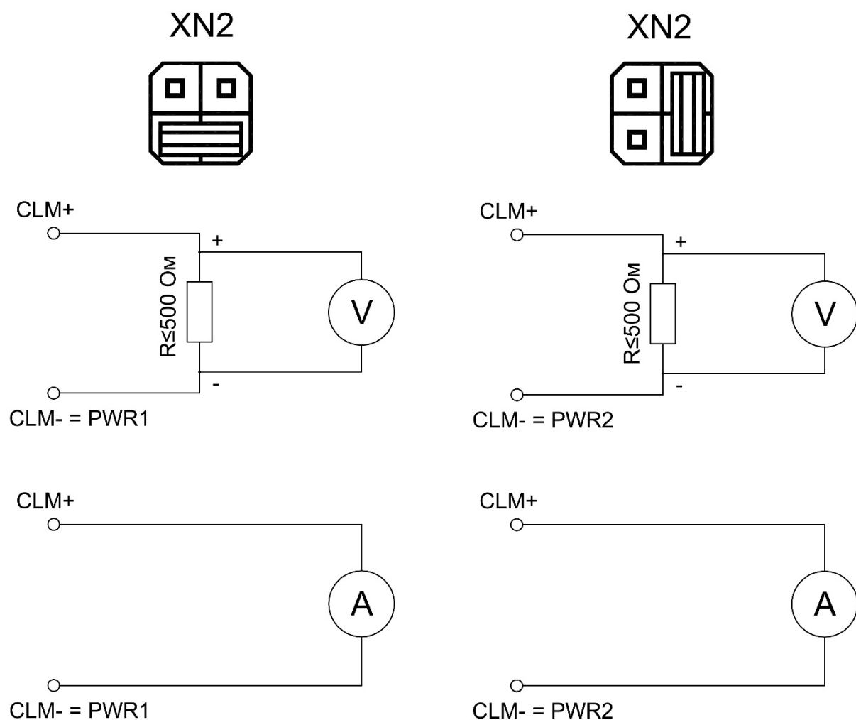
Рисунок Б.2 – Установка перемычки XN2 при подключении по трехпроводной линии: 2 провода питания и один провод CLM+ (активная токовая петля). Заводская установка перемычек: XN2 CLM-=PWR2, XN1 RS 485 LOAD disable.
